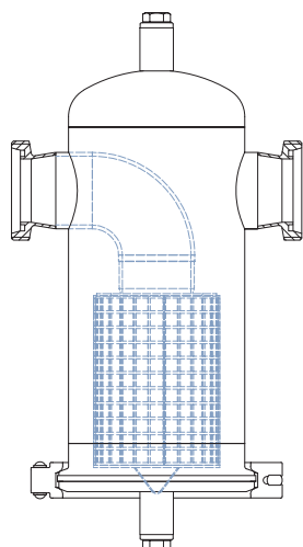
Topfschmutzfänger mit Milchrührverschraubung gemäß DIN 11851 Typ PSA, DN50 PN10
